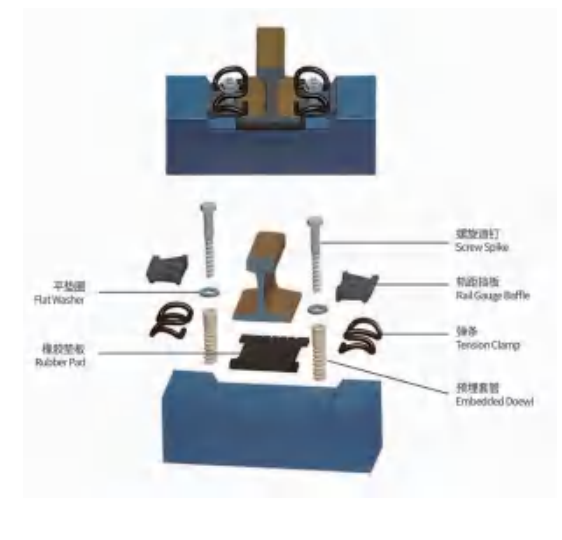
Type V Fastening System 弹条 V 型扣件系统
