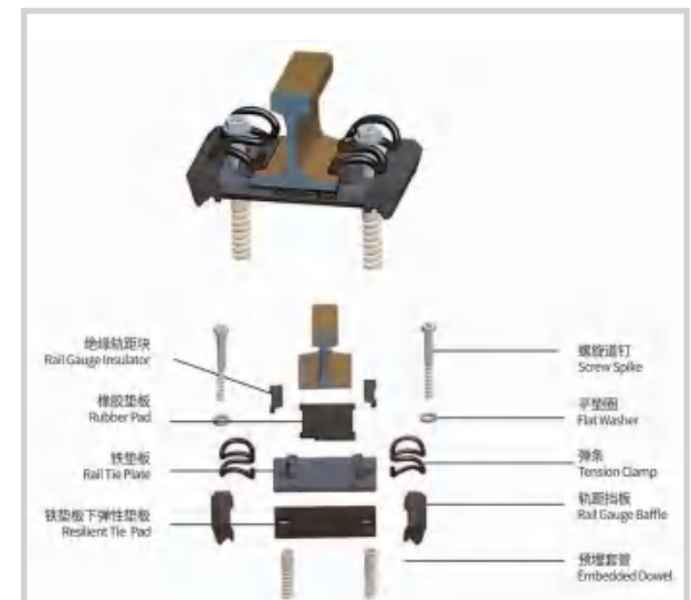
WJ-8 Fastening System WJ-8 型扣件系统
