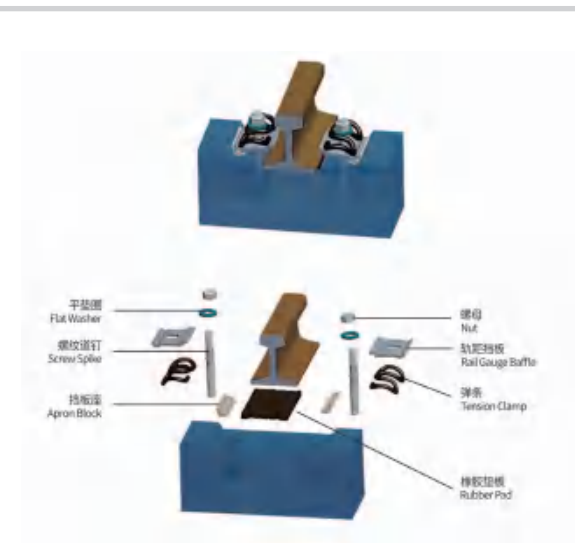
Type II Fastening System 弹条 II 型扣件系统
