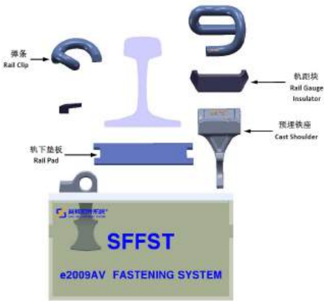
e2009AV Fastening System
