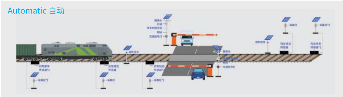
Level Crossing Barriers 平交道口道闸
